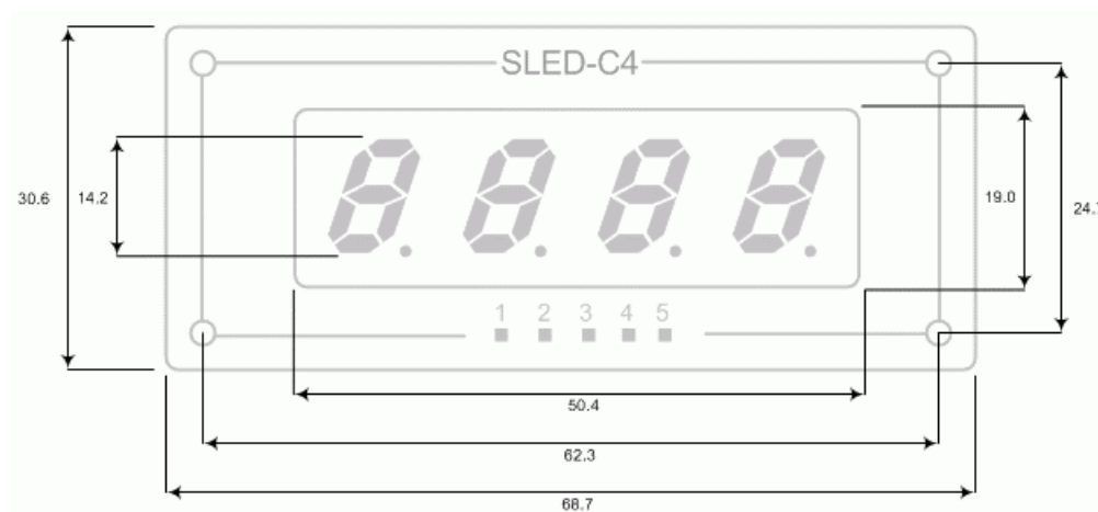
SLED-C4 Dimensions
