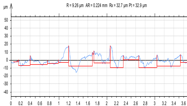
Fig. 14 V=565.74m/min,F=32mm/min.,D=0.75mm
