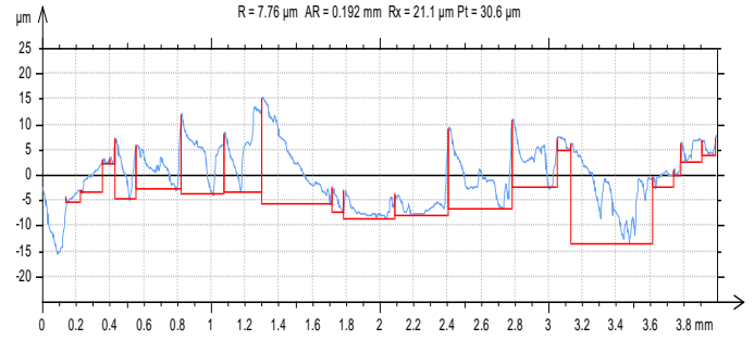
Fig. 23 V=565.74m/min,F=32mm/min.,D=1.00mm
