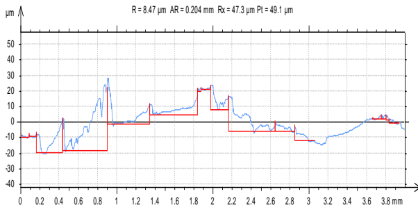
Fig. 12 V=1089.573m/min,F=45mm/min.,D=0.5mm
