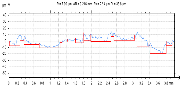
Fig. 13 V=565.74 m/min,F=20mm/min.,D=0.75mm
