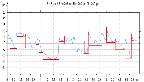
Fig. 20 V=1089.573m/min,F=32mm/min.,D=0.75mm
