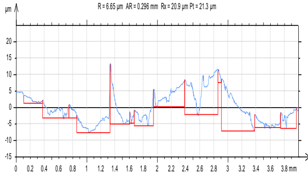
Fig. 19 V=1089.573m/min,F=20mm/min.,D=0.75mm
