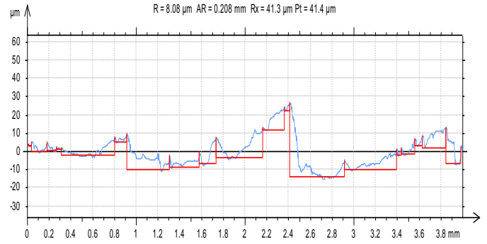
Fig. 15 V=565.74m/min,F=45mm/min.,D=0.75mm
