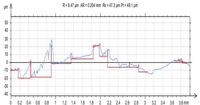
Fig. 10 V=1089.573m/min, F=20mm/min., D=0.5mm
