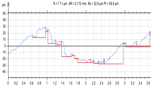
Fig. 29. V=1089.573m/min, F=32mm/min., D=1.00mm
