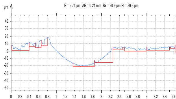
Fig. 6 V=565.74m/min, F=45mm/min., D=0.5mm
