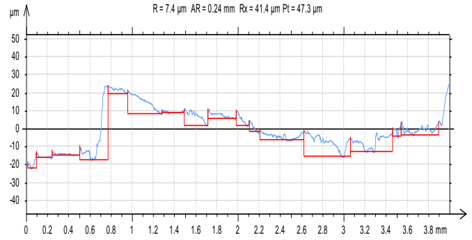
Fig. 7 V=775.273m/min, F=20mm/min, D=0.5mm
