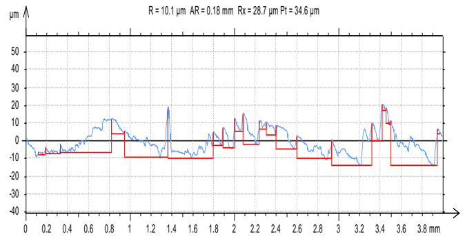
Fig. 17 V=775.273m/min,F=32mm/min.,D=0.75mm
