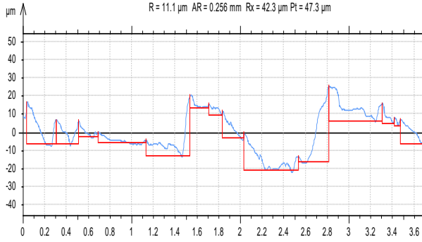
Fig. 28. V=1089.573m/min, F=20mm/min., D=1.00mm
