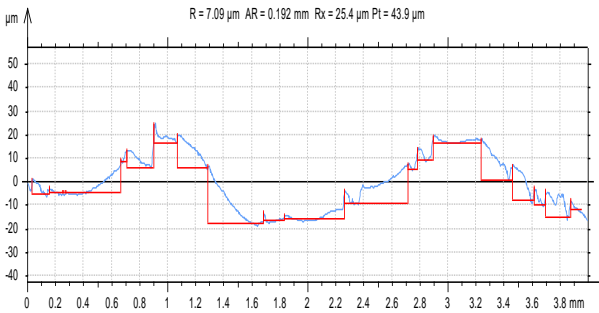
Fig. 30. V=1089.573m/min, F=45mm/min., D=1.00mm
