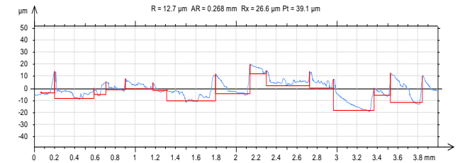
Fig.24.V=565.74m/min,F=45mm/min.,D=1.00mm
