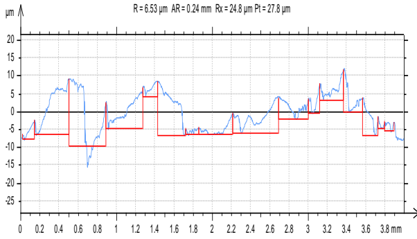
Fig. 11 V=1089.573m/min,F=32mm/min.,D=0.5mm
