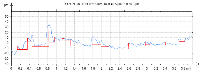
Fig.24.V=565.74m/min,F=45mm/min.,D=1.00mm
