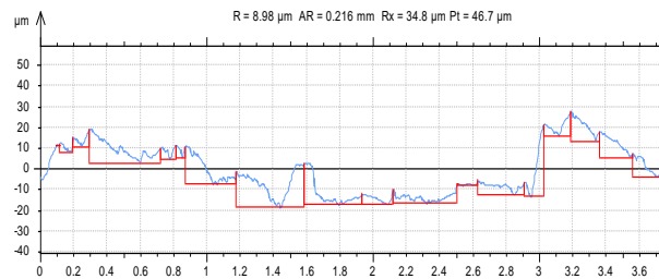
Fig. 22 V=565.74m/min,F=20mm/min.,D=1.00mm
