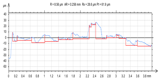
Fig. 27.V=775.273m/min,F=45mm/min.,D=1.00mm
