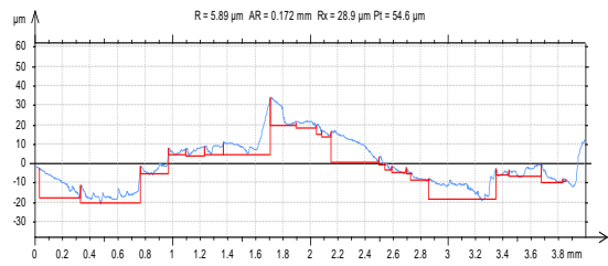
Fig. 5 V=565.74m/min, F=32mm/min., D=0.5mm
