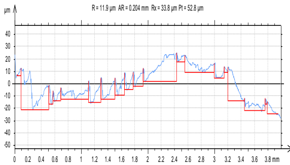
Fig. 4 V=565.74m/min, F=20mm/min., D=0.5mm
