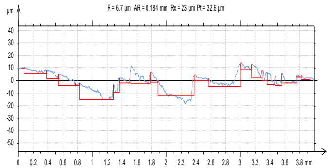
Fig. 8 V=775.273m/min, F=32mm/min., D=0.5mm
