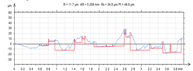
Fig. 26.V=775.273m/min,F=32mm/min.,D=1.00mm
