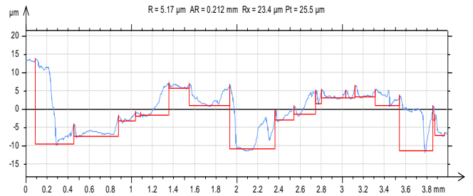
Fig. 16 V=775.273m/min,F=20mm/min.,D=0.75mm
