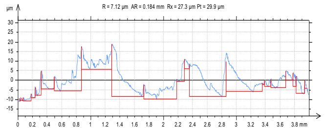
Fig. 9 V=775.273m/min, F=45mm/min., D=0.5mm
