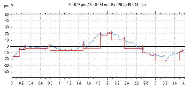
Fig. 21 V=1089.573m/min,F=45M/MIN.,D=0.75MM
