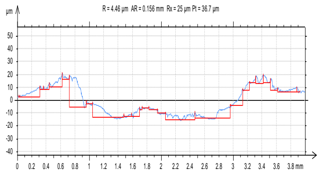
Fig. 18 V=775.273m/min,F=45mm/min.,D=0.75mm
