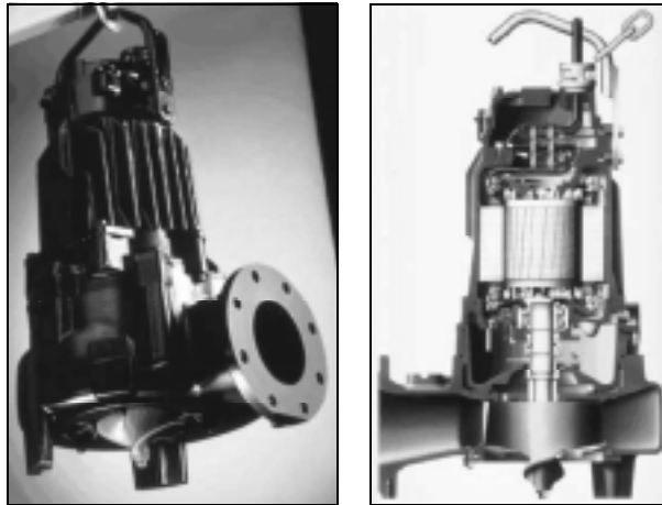
Abb. 3-18: Tauchpumpe mit Schneidkanten am Rotor als Beispiel der Einheit aus Zerkleinerungs- und Förderaggregat Fotos: ITT FLYGT Pumpen GmbH
