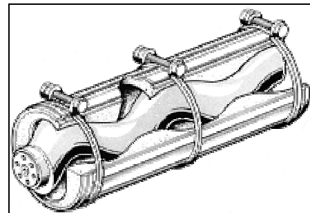
Abb. 3-21: Exzentrerschneckenpumpe (links), nachstellbarer Stator (rechts); Bilder: Armatec-FTS-Armaturen GmbH & Co. KG
