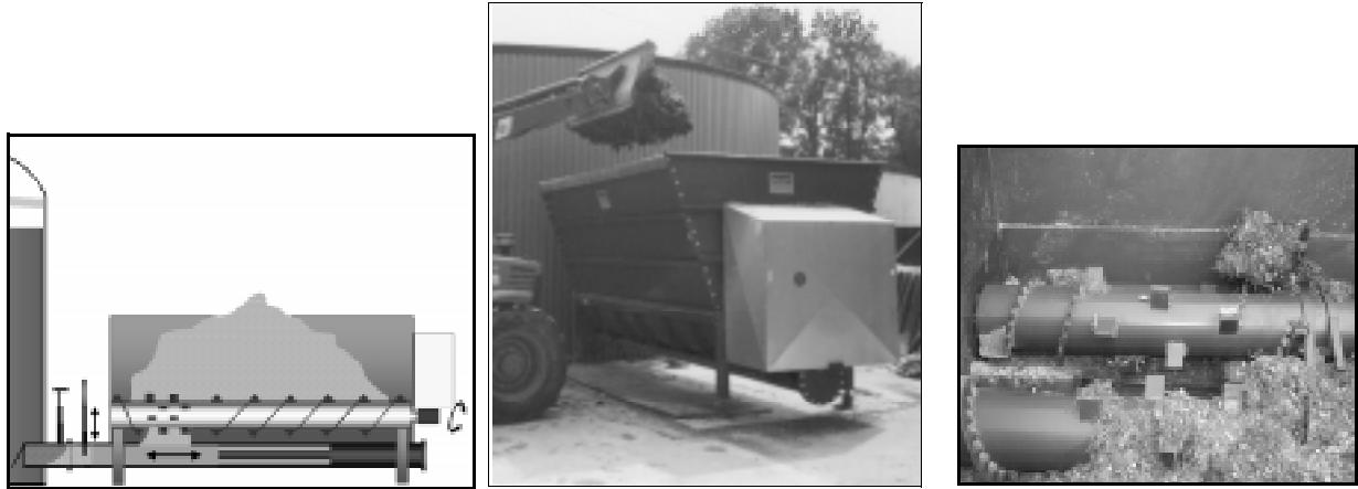
Abb. 3-26: Einbringung stapelbarer Biomasse mit Eintragskolben; Foto: PlanET Energietechnik
