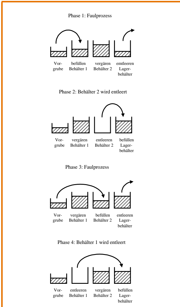
Abb. 3-2: Wechselbehälter-Verfahren
