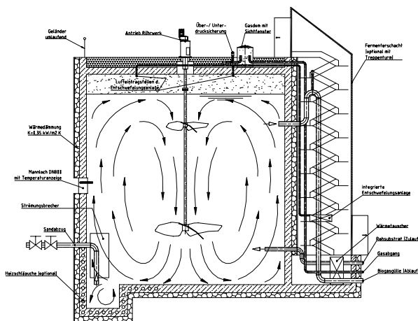
Abb. 3-38: Axialrührwerk; Zeichnung: ENTEC Environmental Technology Umwelttechnik GmbH
