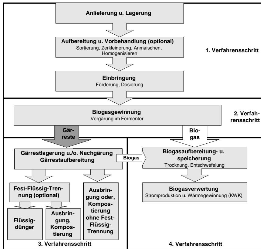
Abb. 3-14: Allgemeiner Verfahrensablauf bei der Biogasgewinnung; nach /3-3/
