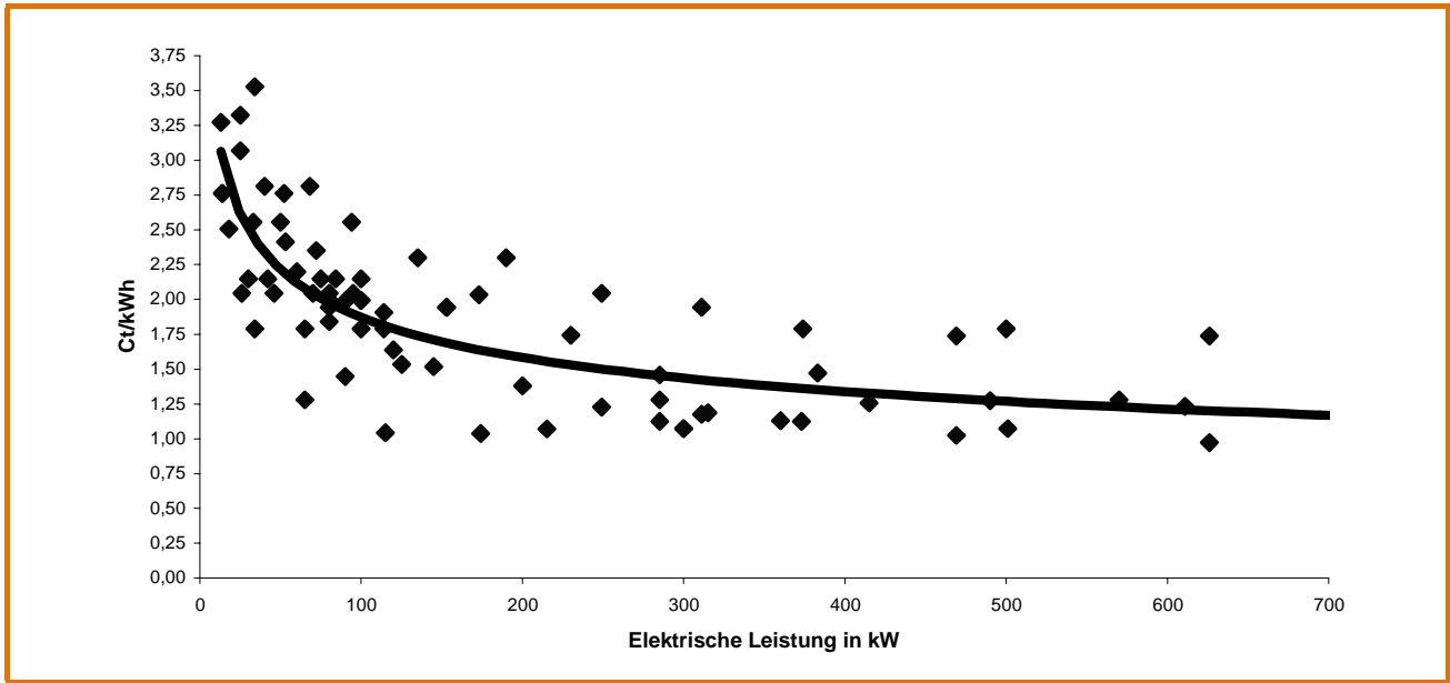
Abb. 5-10: Richtpreise für Instandhaltungsverträge /5-12/
