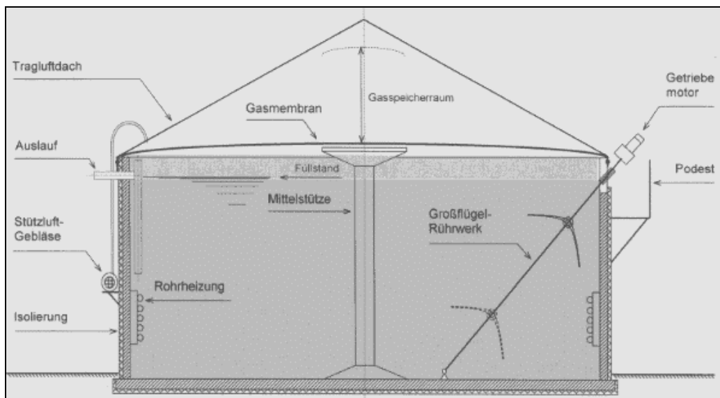
Abb. 3-32: Stehender Fermenter mit Einbauten; Bild: Anlagen- und Apparatebau Lütke GmbH
