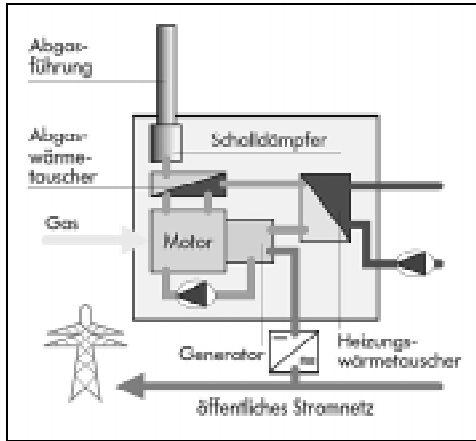
Abb. 5-3: Schematischer Aufbau eines BHKW; Schema: ASUE
