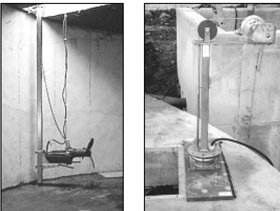
Abb. 3-36: Tauchmotor-Propellerrührwerk (links) und Führungsrohrsystem (rechts); Fotos: Agrartechnik Lothar Becker
