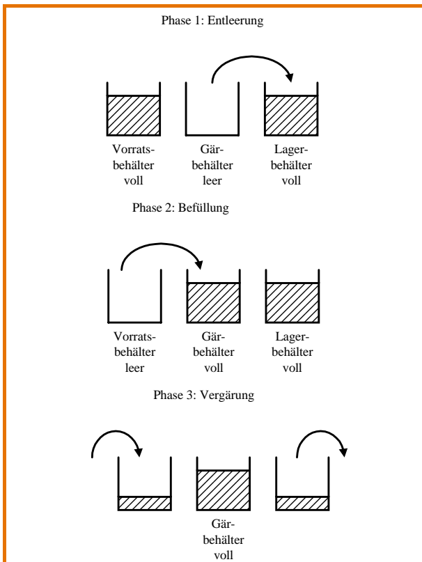
Abb. 3-1: Batchverfahren
