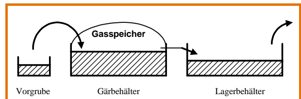
Abb. 3-3: Durchfluss-Verfahren
