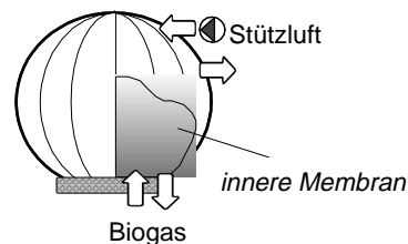
Doppelmembranspeicher
