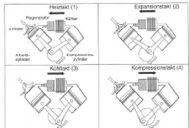
Abb. 5-11: Arbeitsweise eines Stirlingmotors aus /5-14/ nach /5-24/
