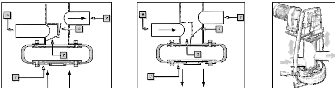
Abb. 3-23: Funktionsprinzip Balgpumpe (Flansch (1), Ventile (2 und 3), Auslass (4), Einlass (5)) Bilder: Armatec-FTS-Armaturen GmbH & Co. KG
