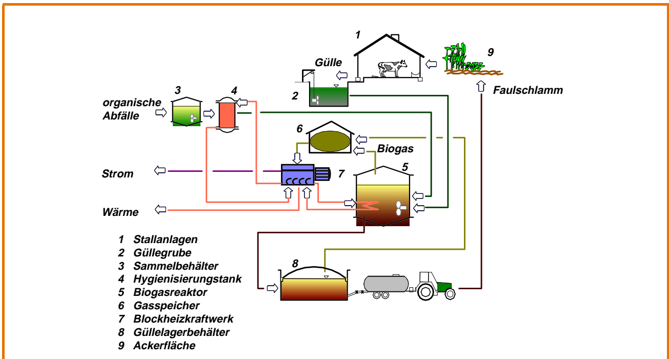
Abb. 3-15: Schema einer landwirtschaftlichen Biogasanlage mit Verwendung von Kosubstraten; Schema: B. Linke, Institut für Agrartechnik Bornim
