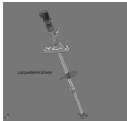
Abb. 3-37: Langachsrührwerke mit zwei Rührwerkzeugen mit und ohne Lagerung am Fermenterboden; Foto: WELtec BioPower GmbH; Grafik: Armatec FTS-Armaturen GmbH & Co. KG
