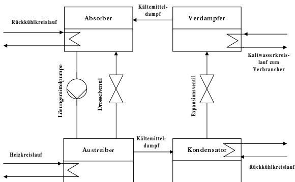
Abb. 5-14: Funktionsschema einer Absorptionskältemaschine
