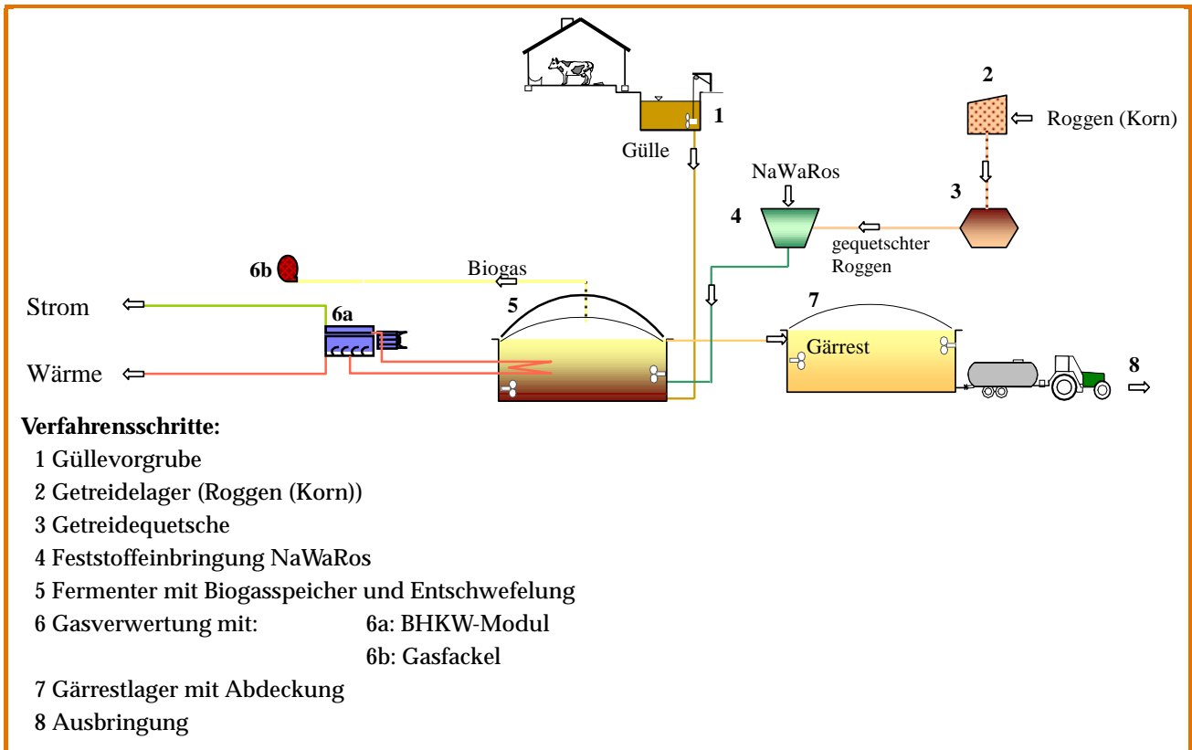
Abb. 6-3: Verfahrensfließbild der Modellanlage 2
