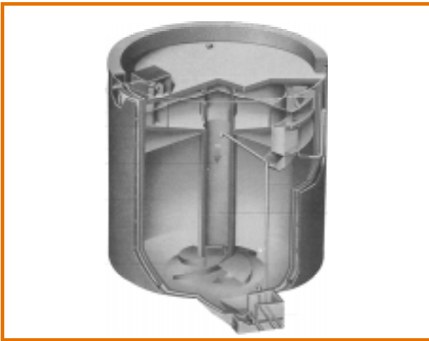
Abb. 3-8: Doppelkammer-Fermenter; Abbildung: ENTEC Environment Technology Umwelttechnik GmbH
