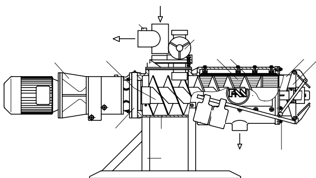
Abb. 3-40: Schneckenseparator; Zeichnung: FAN Separator GmbH; Foto: PlanET Energietechnik
