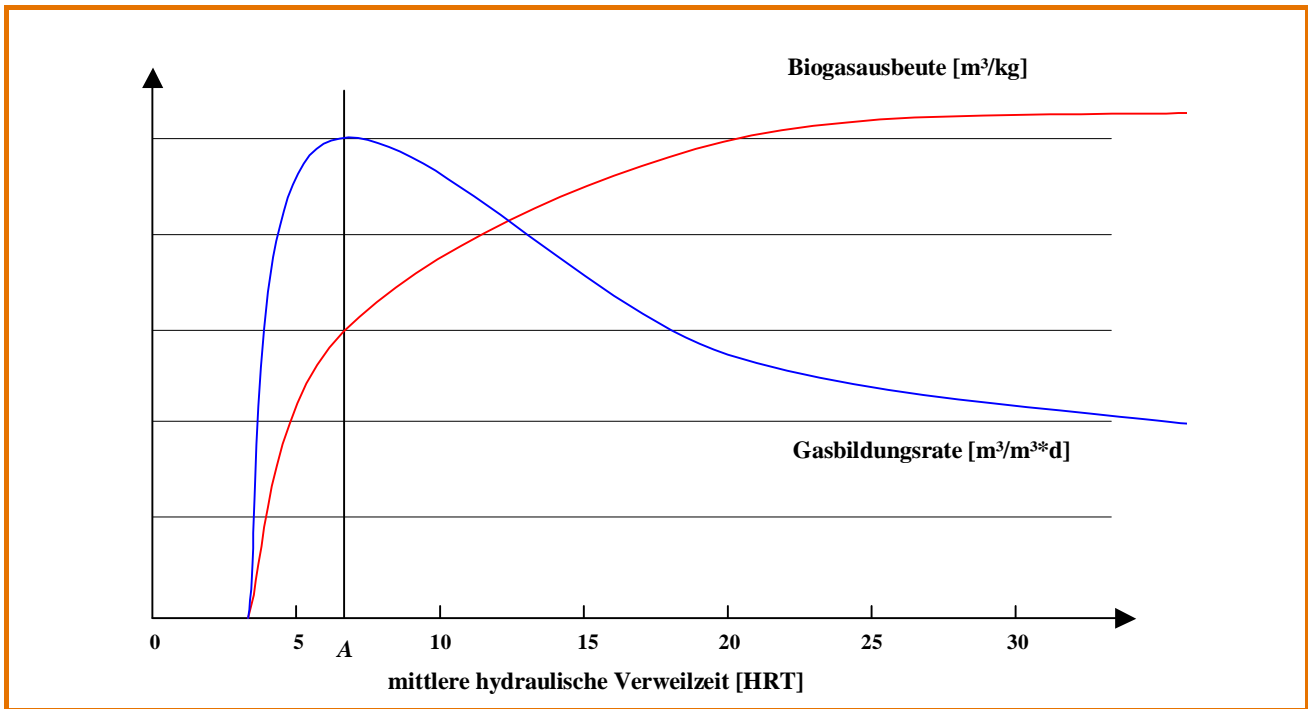
Abb. 2-4: Biogasausbeute und Gasbildungsrate in Abhängigkeit von der Verweilzeit (nach/2-12/)
