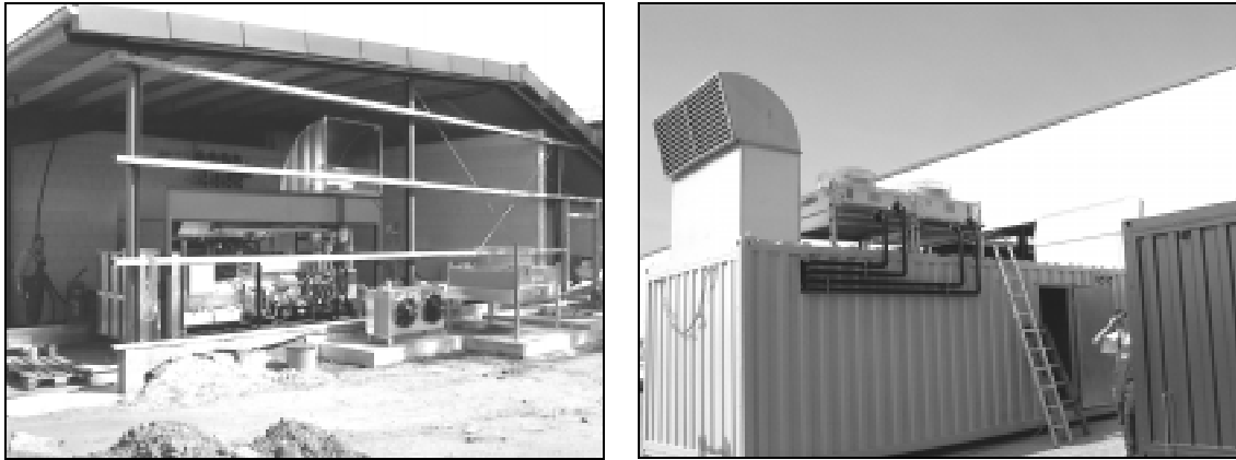
Abb. 5-8: BHKW-Container bzw. Aufbau eines BHKW in einem Gebäude; Fotos: Seva Energie AG
