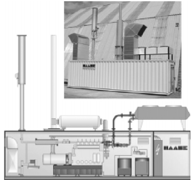
Abb. 5-4: Biogas-BHKW, Komplettmodul in Kompaktbauweise mit Notfackel; Abb.: Haase Energietechnik AG
