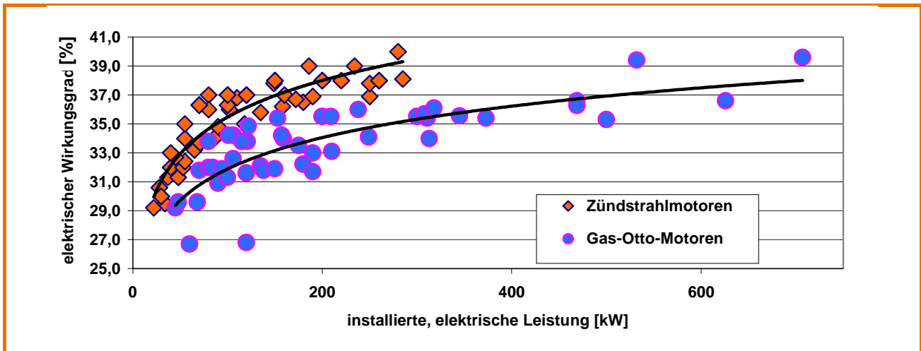
Abb. 5-5: Elektrischer Wirkungsgrad von Biogas-BHKW nach Herstellerangaben; nach /5-25/, erweitert
