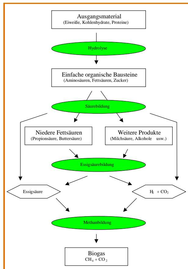
Abb. 2-1: Schematische Darstellung des anaeroben Abbaus
