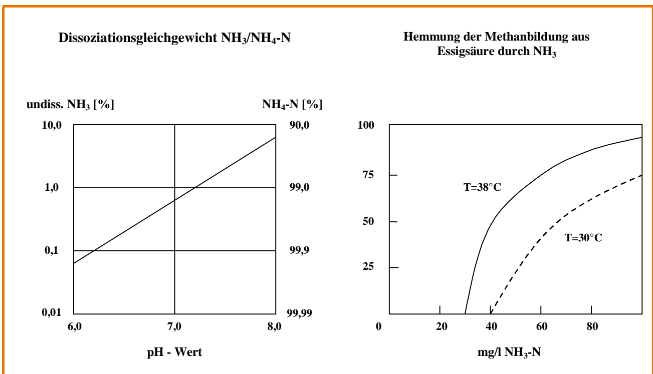
Abb. 2-2: Hemmung der Methanbildung aus Essigsäure durch \text{NH}_3 (nach /2-11/)
