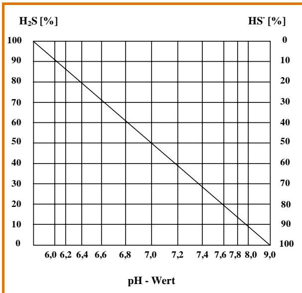
Abb. 2-3: Anteil von HS - und H 2 S in Abhängigkeit vom pH-Wert (nach /2-11/)
