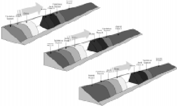
Abb. 3-12: Kombinierte Trockenfermentation mit dem 3-A-Verfahren, schematisch; Abbildung: S.I.G. - Dr.-Ing. Steffen GmbH
