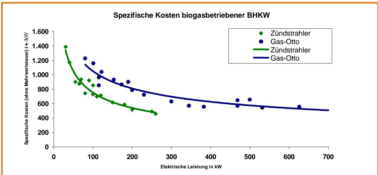
Abb. 5-9: Spezifische Kosten von Biogas-BHKW
