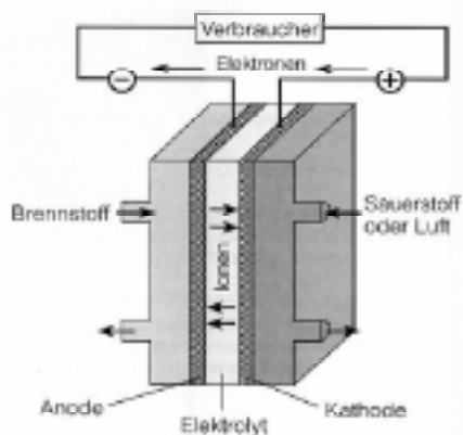
Abb. 5-13: Funktionsprinzip einer Brennstoffzelle; Zeichnung: FAL Braunschweig
