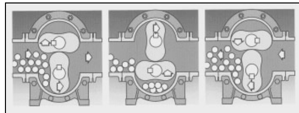
Abb. 3-22: Drehkolben-Pumpprinzip; Bild: Vogelsang GmbH
