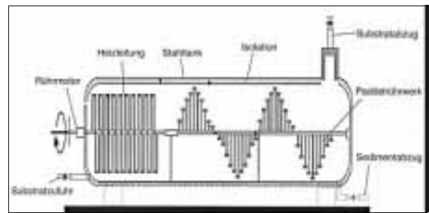
Abb. 3-31: Liegender Tankfermenter mit Paddelrührwerk /3-4/
