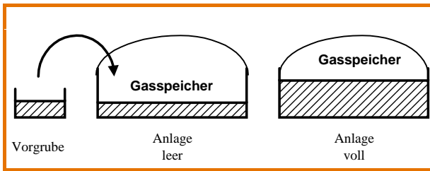
Abb. 3-4: Speicher-Verfahren
