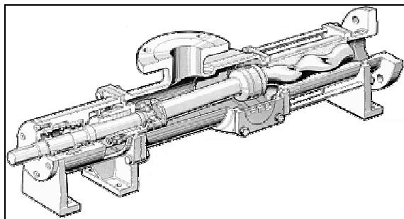
Abb. 3-21: Exzentrerschneckenpumpe (links), nachstellbarer Stator (rechts); Bilder: Armatec-FTS-Armaturen GmbH & Co. KG
