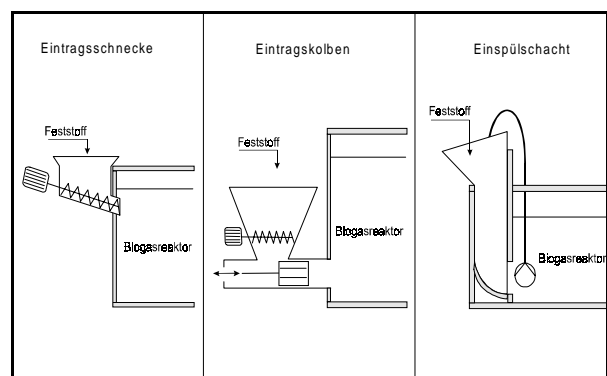
Abb. 3-25: Verfahren zur Einbringung stapelbarer Biomasse; Bild: FAL Braunschweig
