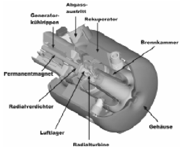
Abb. 5-12: Aufbau einer Mikrogasturbine; Bild: G.A.S. Energietechnologie GmbH
