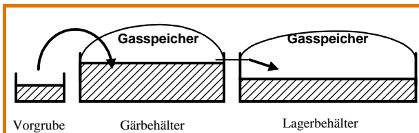
Abb. 3-5: Kombiniertes Durchfluss-Speicher-Verfahren
