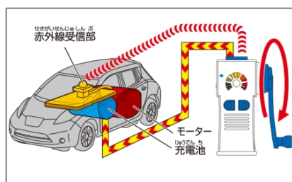
左図： 発電の仕組み
