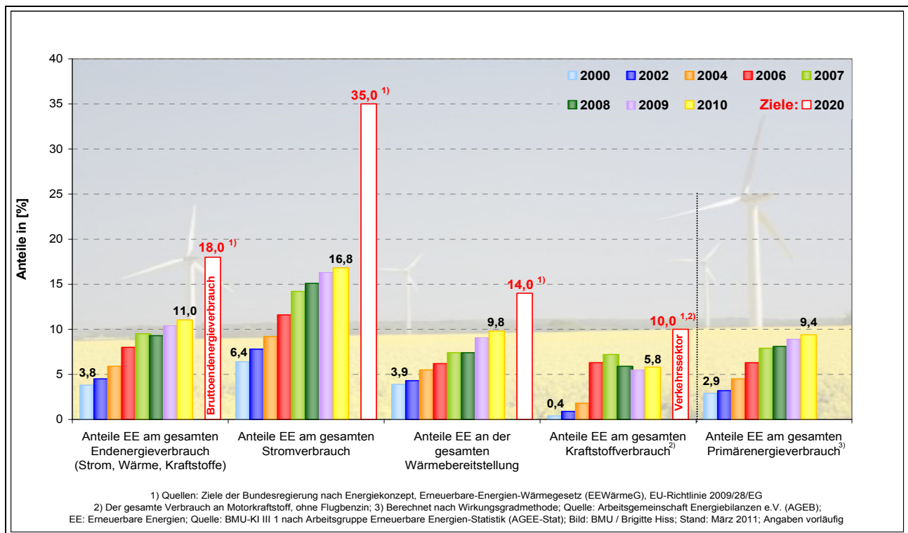
Abb. 2: Anteile erneuerbarer Energien an der Energiebereitstellung in Deutschland
