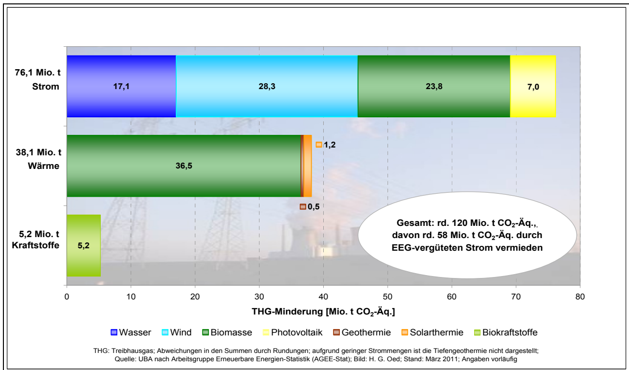
Abb. 3: Vermiedene Treibhausgas-Emissionen durch die Nutzung erneuerbarer Energien in Deutschland - 2010
