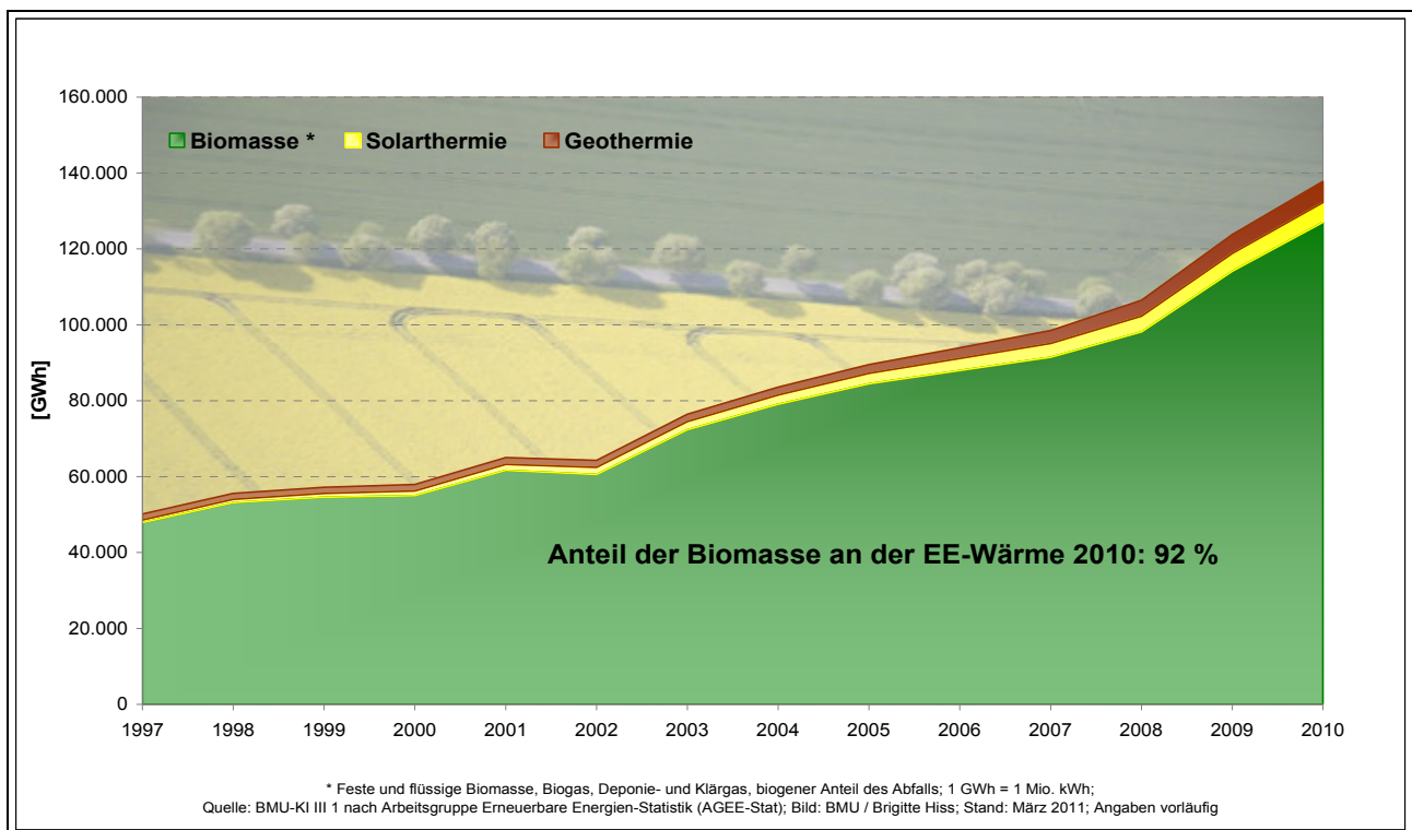
Abb. 6: Wärmebereitstellung aus erneuerbaren Energien in Deutschland 1997 bis 2010
