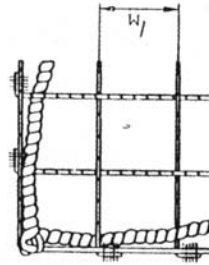
a) quadratische Masche (Q)
