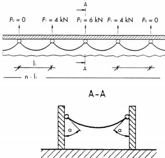
Bild 7: Beispiel für charakteristische Lasten an den Aufhängepunkten
