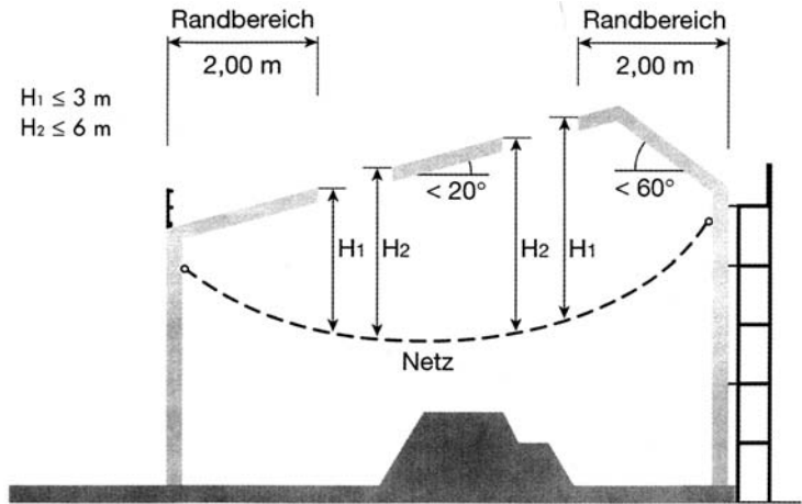
Bild 5: Zulässige Absturzhöhen für System S
