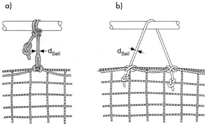
Bild 6: Beispiele für Netzaufhängungen durch Umschlingung und Verknotung mit
