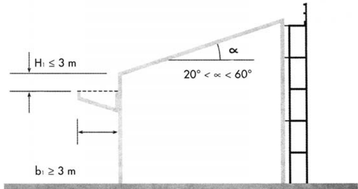
Bild 11: Zulässige Absturzhöhen und erforderliche Fangbreiten bei > 20^\circ geneigten Flächen
