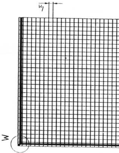
a) quadratische Masche (Q)
