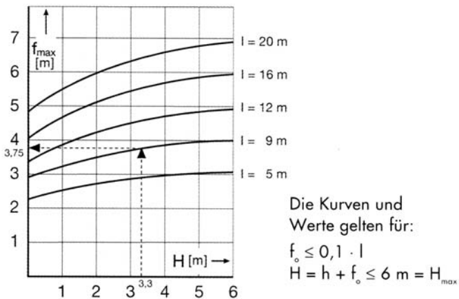
Bild 9: Verformungen des Schutznetzes in Abhängigkeit von der Spannweite und Lage der Aufhängungspunkte
