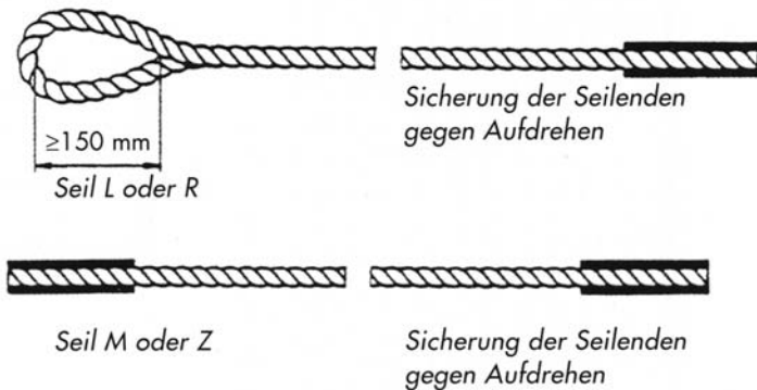
Bild 3: Beispiele für Aufhängeseile
