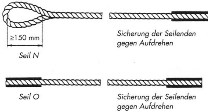
Bild 4: Beispiele für Kopplungsseile
