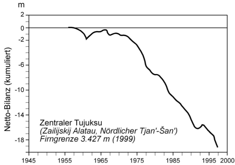
Abb. 11: Entwicklung der Netto-Massenbilanz von Gletschern im Tjan'-Šan' 1945-2000
