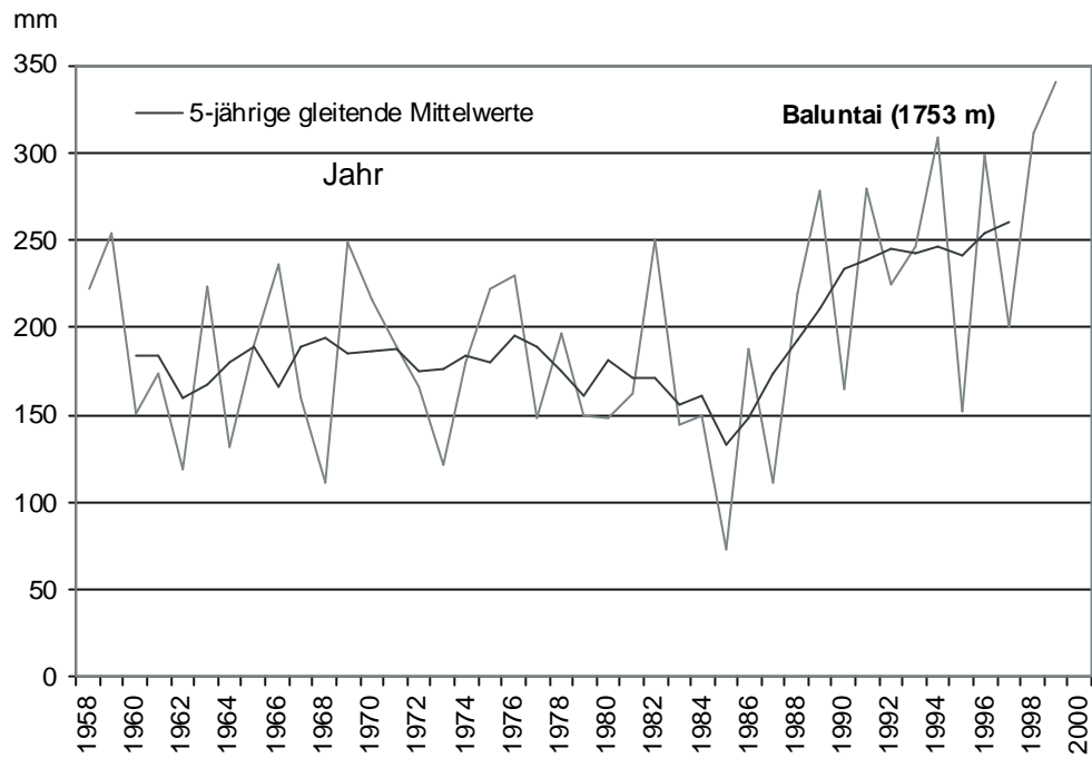
Abb. 9: Entwicklung der jährlichen und sommerlichen Niederschlagsmengen der Station Baluntai 1958 - 2000
