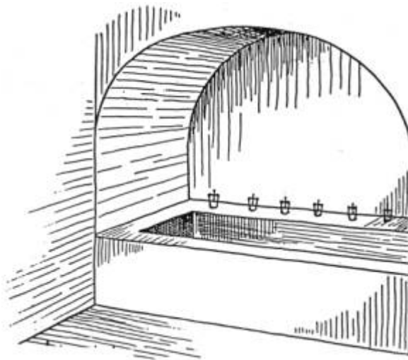
Abb. 13: Arcosol-Troggrab.
