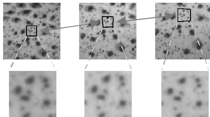
Abb. 1: Objektaufnahmen zu drei verschiedenen Zeitpunkten bzw. Verformungszuständen. Das Muster im Subset wird verschoben und gedehnt.
