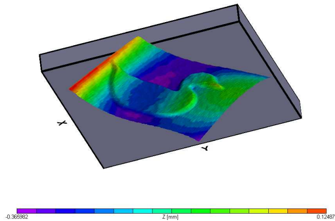
Abb. 7: Konturmessung: Papierdicke Ente auf einer leicht gebogenen Plexiglasscheibe.
