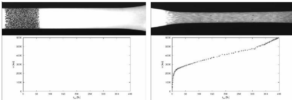
Abb. 3: Erstes und letztes Bild einer automatisch ausgewertete Bildsequenz: Zugprobe aus HDPE mit einer Dehnung bis 400%.
