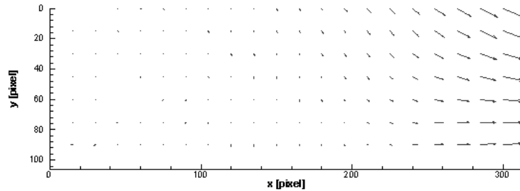
Abb. 2: Das Verschiebungsvektorfeld einer Zugprobe die horizontal gedehnt wurde. Die Vektoren auf der rechten Seite verdeutlichen das Einschnüren der Probe.
