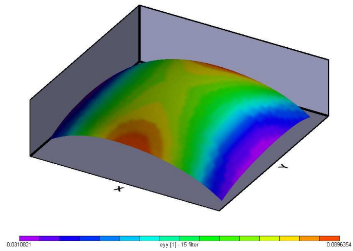
Abb. 9: Dehnungsbestimmung bei einer Gummimembran.
