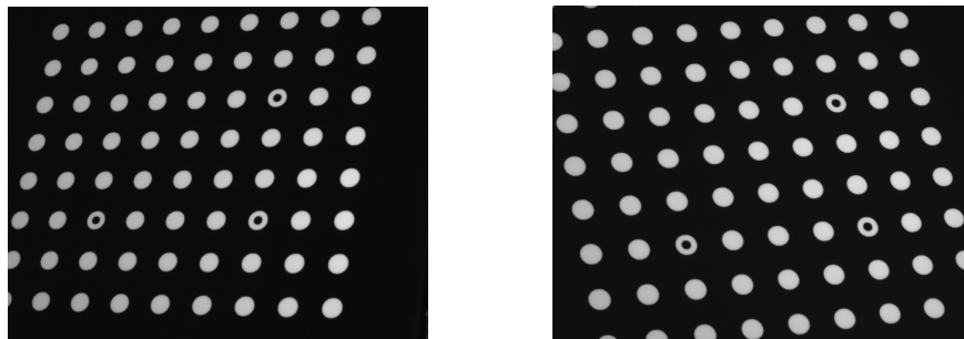
Abb. 5: Linkes und rechtes Kamerabild des Kalibrierobjektes.
