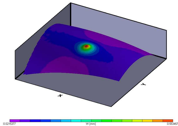
Abb. 8: Verschiebungsbestimmung: Steinschlagdelle in einem KFZ-Blech.
