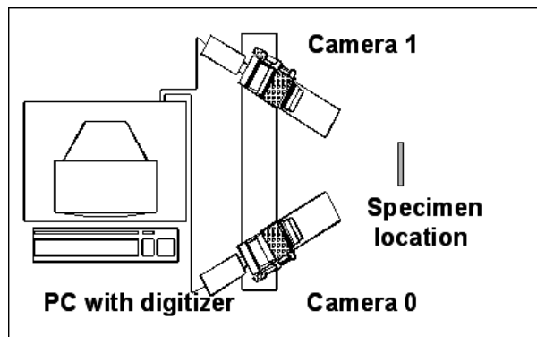
Abb. 4: Stereoskopisches Prinzip zur 3D-Verformungsmessung bestehend aus 2 Kameras mit unterschiedlichen Orientierungen.
