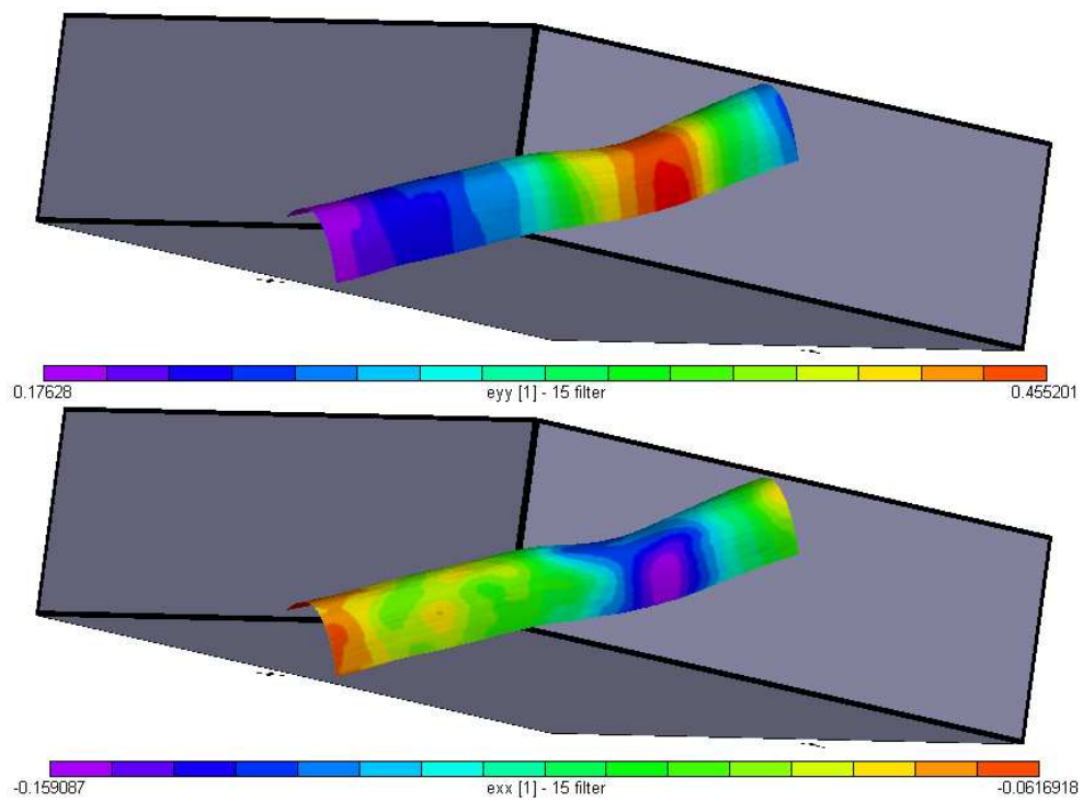
Abb. 10: Dehnungsbestimmung bei einer Zugprobe aus Stahl.
